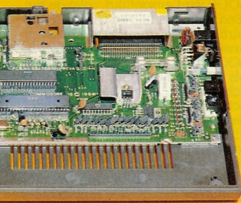
Im Gehäuse ist noch viel Platz
